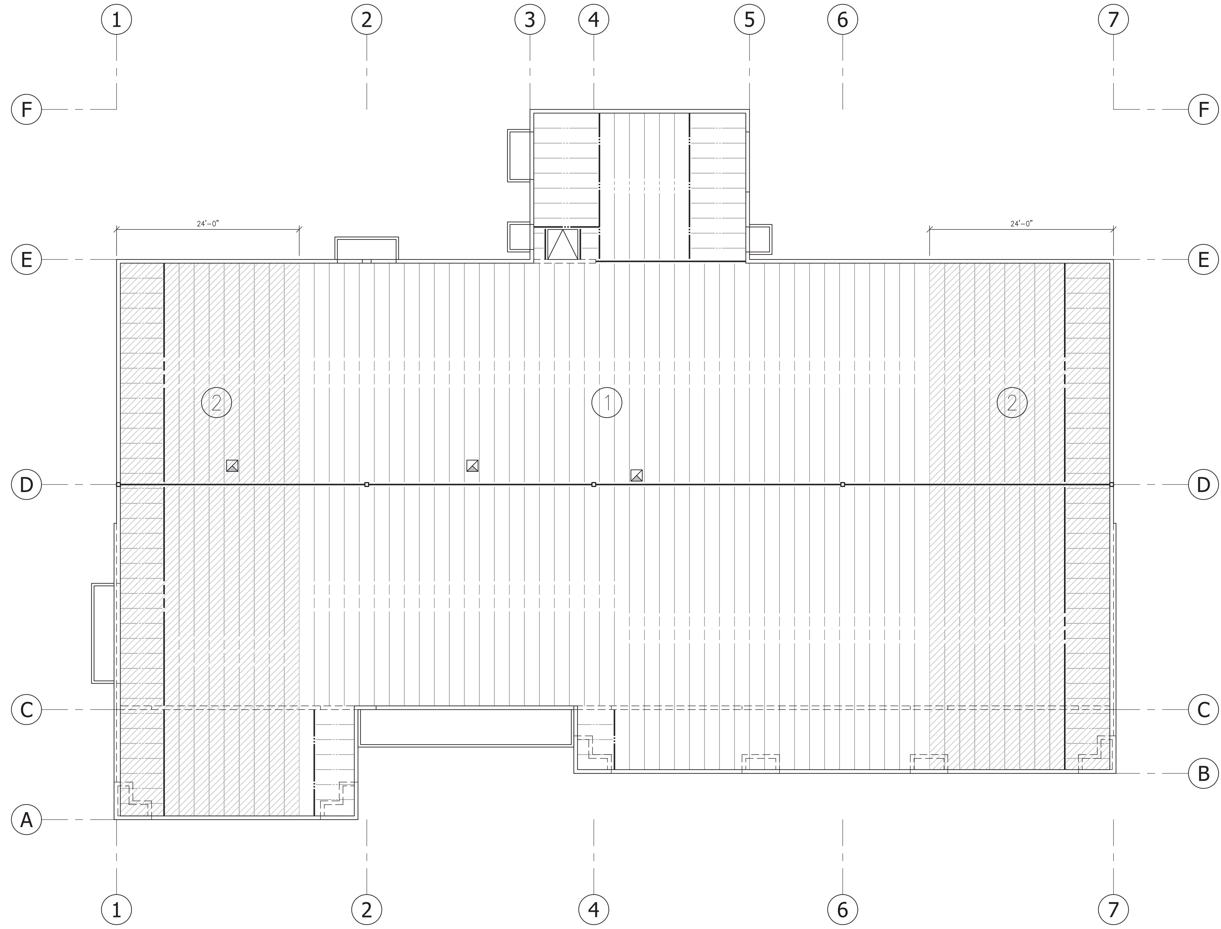
NAILING PLAN SCALE: 1/8" = 1'-0"
